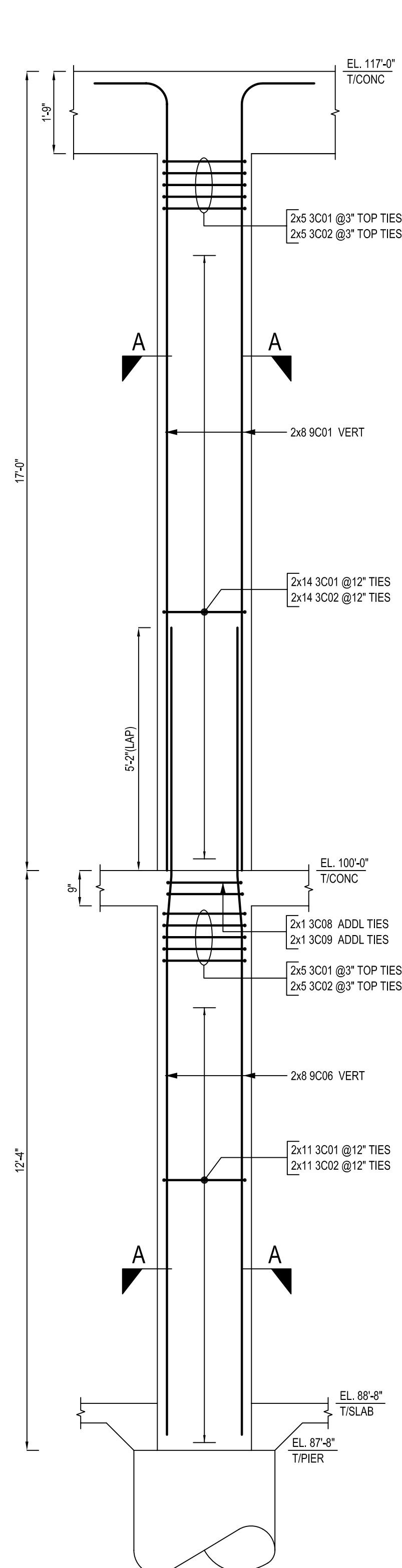
COLUMN - C1l SCALE: 1/2"=1'-0" SDR: 12/S-201 & S-311 (2 LOC)
