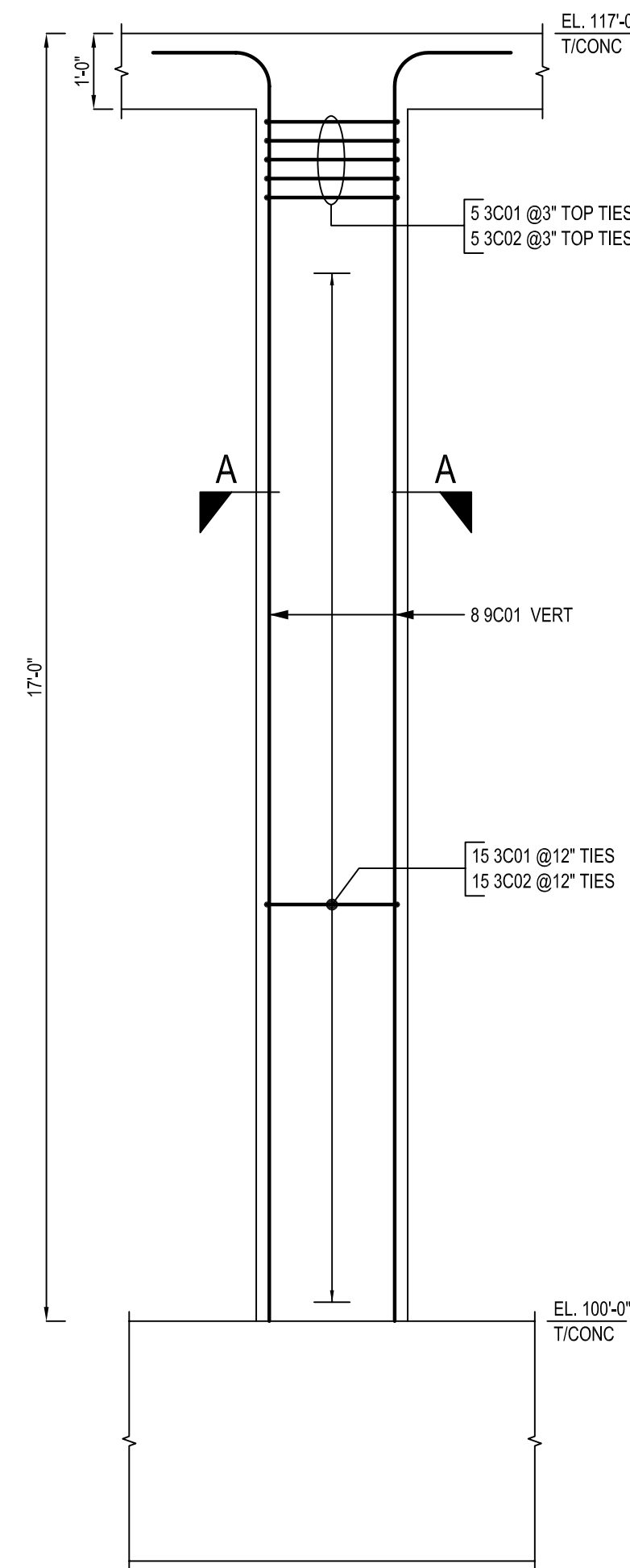
COLUMN - C2a SCALE: 1/2"=1'-0" SDR: 12/S-201 & S-311 (1 LOC)
