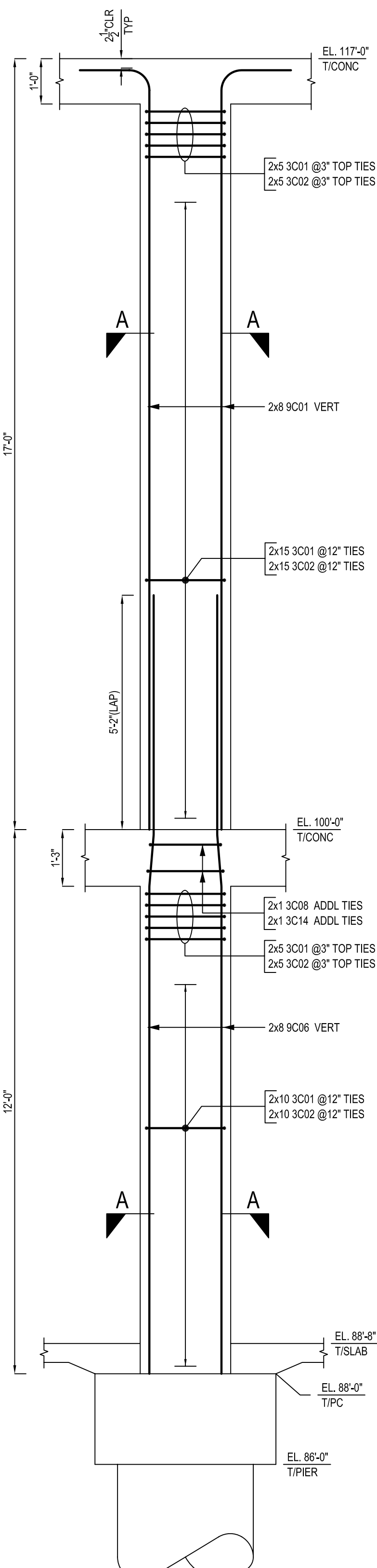
COLUMN - C1h SCALE: 1/2"=1'-0" SDR: 12/S-201 & S-311 (2 LOC)
