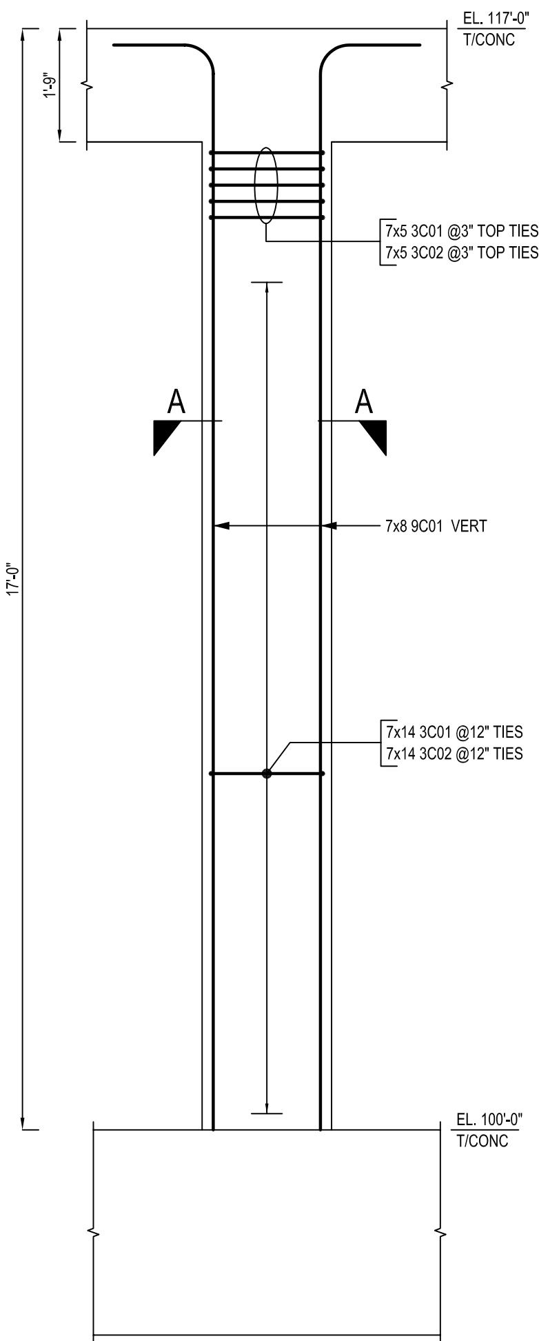
COLUMN - C2 SCALE: 1/2"=1'-0" SDR: 12/S-201 & S-311 (7 LOC)
